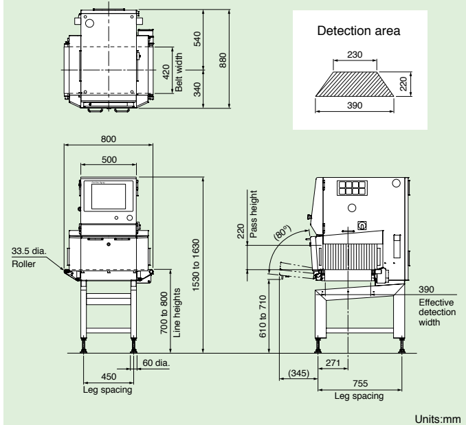
Units:mm
